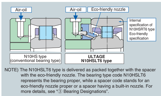
Fig. 10.15 N10HSLT6 type
